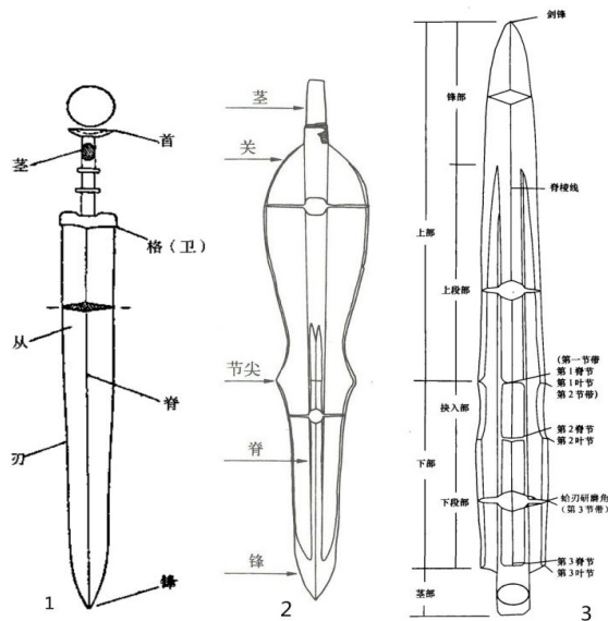
图一 中原式铜剑和短茎铜剑细节名称
