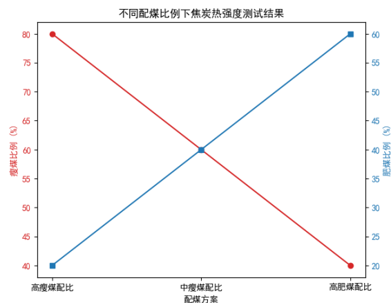
图1 不同配煤比例下焦炭热强度测试结果
