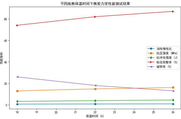
图 2 不同炼焦保温时间下焦炭力学性能测试结果
