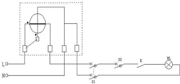
图2 书房一控一灯电路原理图
