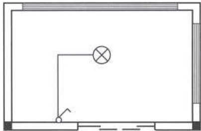
图3 书房一控一灯电路安装平面示意图（施工图）
